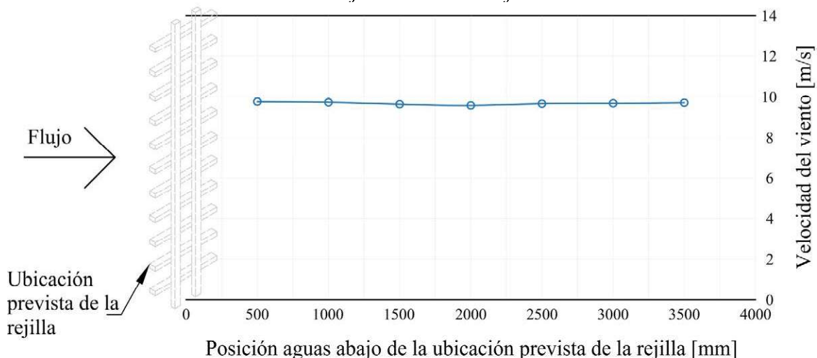
Gráfica 1. Velocidad del viento en el eje del túnel sin rejilla de turbulencia
