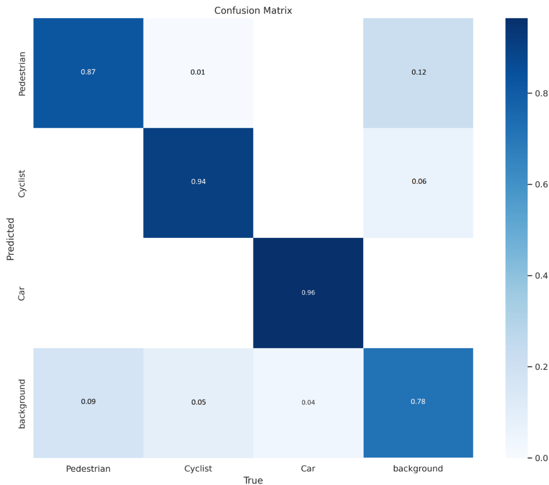
Figura 5. 6 Matriz de confusión para el entrenamiento de la mejor combinación de hiperparámetros para la segunda solución.
