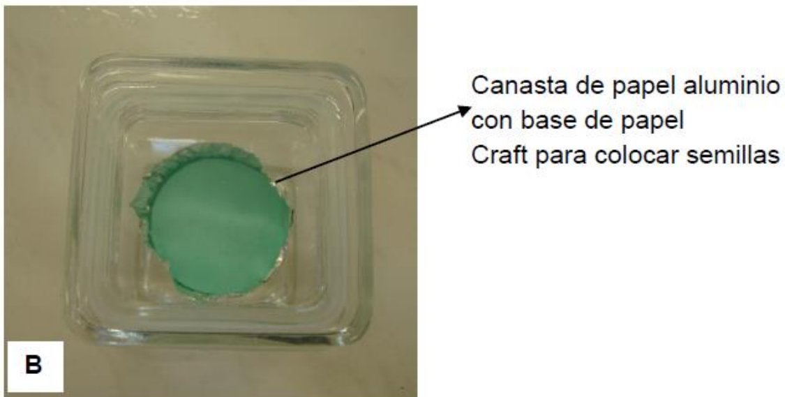
Figura 1. Sistema de deshidratación con tapa separada. A) Vista frontal con sus respectivas partes. B). Vista superior mostrando canasta para colocación de semillas.
