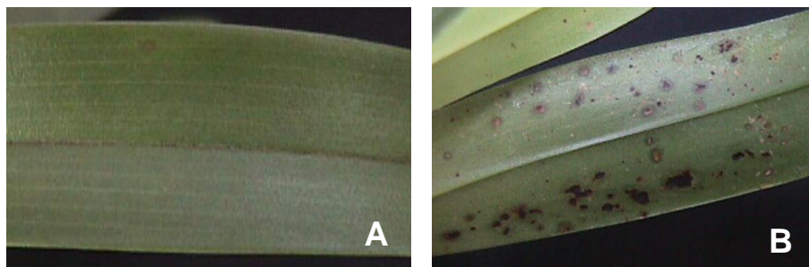
Figura 5. Síntomas foliares presentes en una planta de Maxillaria sp. A. Líneas cloróticas en toda la hoja. B. Zonas necróticas con apariencia a infección fungosa.
