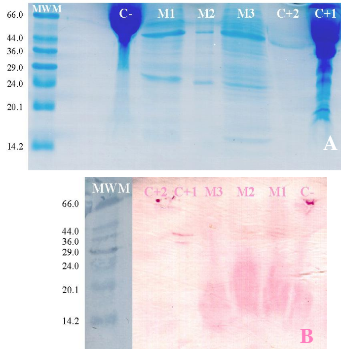
Figura 8. A. Gel desnaturalizante de poliacrilamida (SDS-PAGE) teñido con azul de Coomasie. B. Transferencia a papel de nitrocelulosa del gel par al mostrado en A y revelado con anticuerpo específico para el virus BCMV. MWM= marcadores de peso molecular kDa, C- = control negativo, M1= muestra 1, M2= muestra 2, M3= muestra 3, C+1 = control positivo BCMV, C+2 = control positivo potyvirus.
