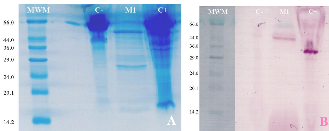
Figura 9. A. Gel desnaturalizante de poliacrilamida (SDS-PAGE) teñido con azul de Coomassie. B. Transferencia a papel de nitrocelulosa del gel par al mostrado en A y revelado con anticuerpo específico para el virus TuMV. MWM= marcadores de peso molecular kDa, C- = control negativo, M1= muestra 1, C+ = control positivo TuMV.
