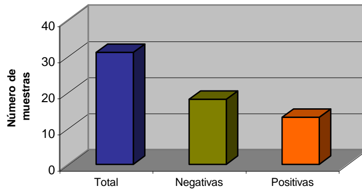
Figura 12. Muestras positivas y negativas para INSV de las 31 orquídeas nativas evaluadas
