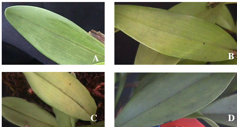
Figura 11. Síntomas más comunes observados en las plantas de orquídeas evaluadas para la detección del virus INSV.
