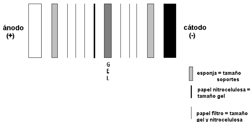
Figura 1.1. Orden de montaje de las partes que componen el “sandwich” requerido para llevar a cabo la transferencia.
