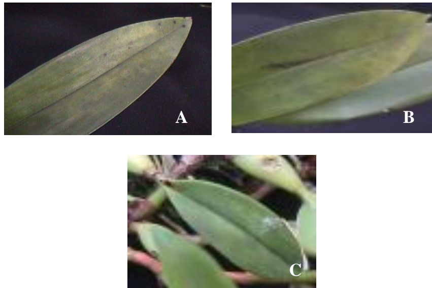
Figura 2. Moteado clorótico presente en plantas de Mesospinidium warscewiczii (A), Maxillaria criptobulbom (B) y Encyclia pigmeae (C).
