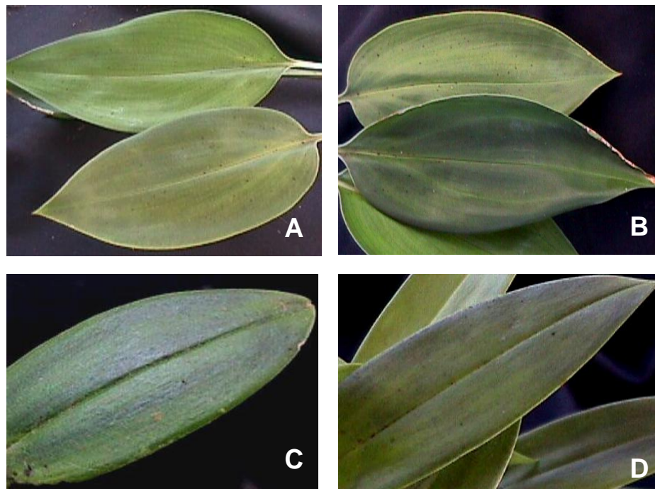
Figura 3. Bandeados observados en algunas muestras evaluadas mediante la técnica de ELISA para la detección de potyvirus. A y B. Bandeados cloróticos y aclaramiento de venas en Prescottia stachyodes . B. Deformación foliar (acucharamiento) en P. stachyodes . C. Bandeado clorótico entre las venas y en el margen de las hojas de Encyclia pigmeae . D. Bandeado clorótico en hojas de Maxillaria ramonensis .
