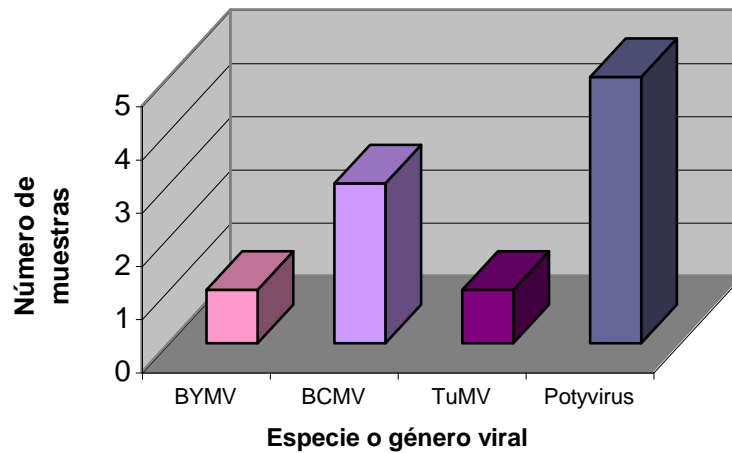
Figura 7: Total de muestras positivas para cada una de las especies evaluadas del género Potyvirus
