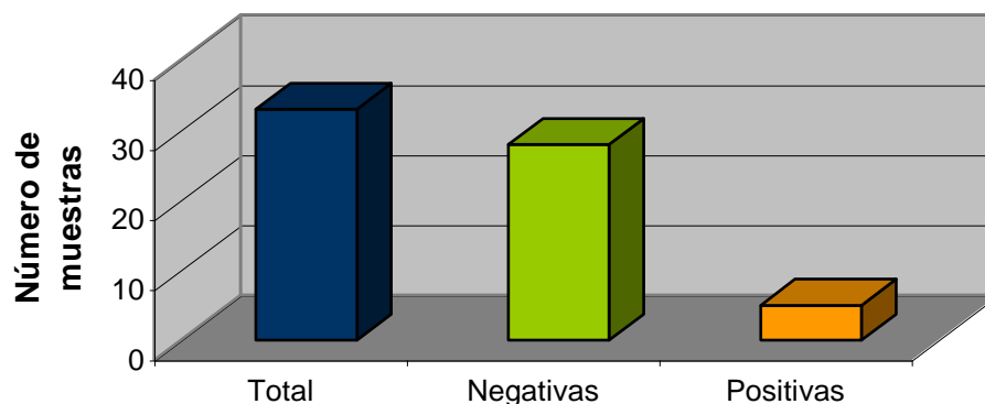
Figura 6. Muestras positivas y negativas para potyvirus de las 33 orquídeas nativas evaluadas
