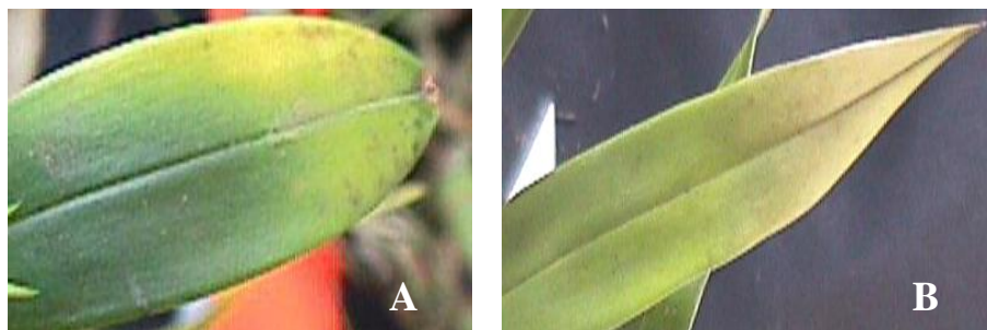
Figura 4. Amarillamiento severo en la región apical y márgenes de la hoja. A. Encyclia pigmeae , B. Maxillaria ramonensis .
