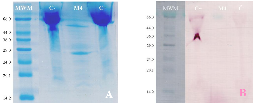
Figura 10. A. Gel desnaturalizante de poliacrilamida (SDS-PAGE) teñido con azul de Coomassie. B. Transferencia a papel de nitrocelulosa del gel par al mostrado en A y revelado con anticuerpo específico para el virus BYMV. MWM= marcadores de peso molecular kDa, C- = control negativo, M4= muestra 04-003, C+ = control positivo BYMV.
