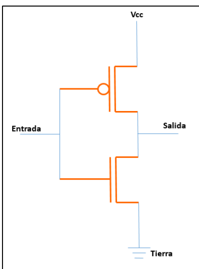
Figura 1: Esquemático de un circuito inversor
