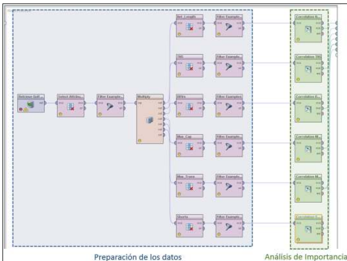
Figura 32: Proceso de análisis de correlación para variables de QoR
