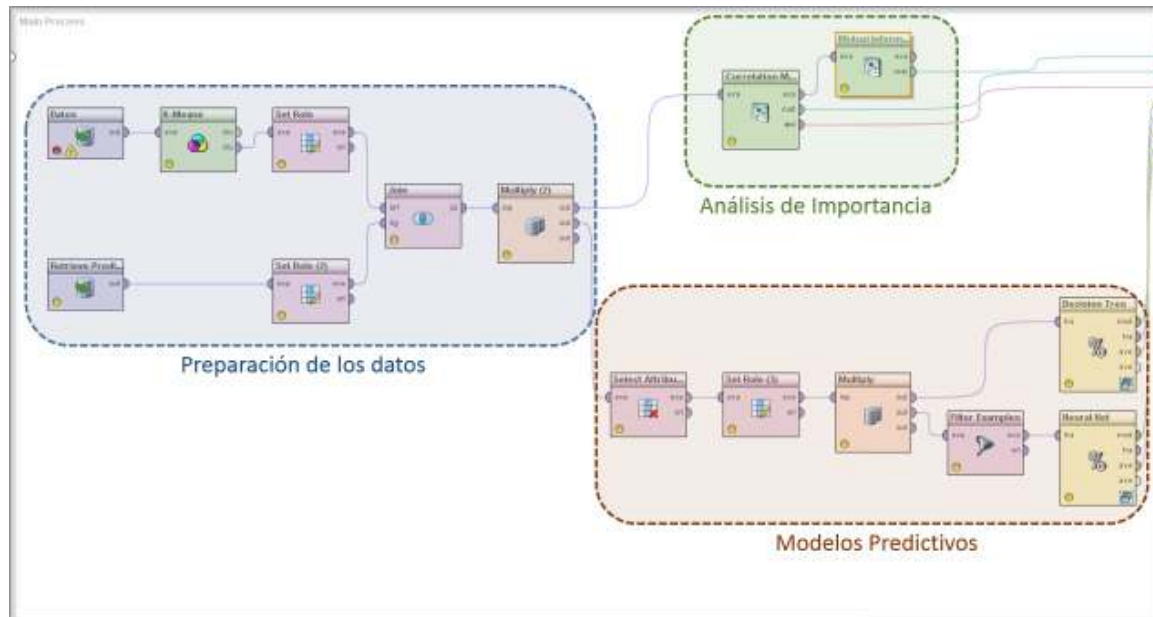
Figura 22: Proceso para generar modelo predictivo de complejidad de particiones
