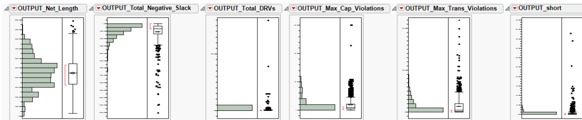
Figura 31: Distribuciones de las variables de QoR
