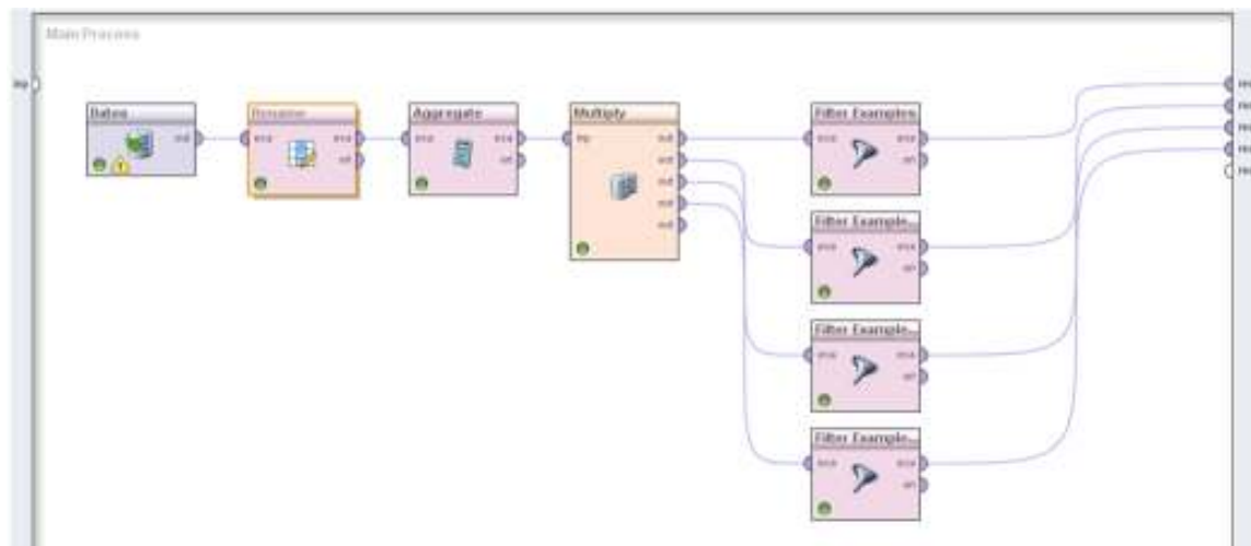
Figura 16: Proceso de RapidMiner para el análisis jerárquico de violaciones de tiempo máximo
