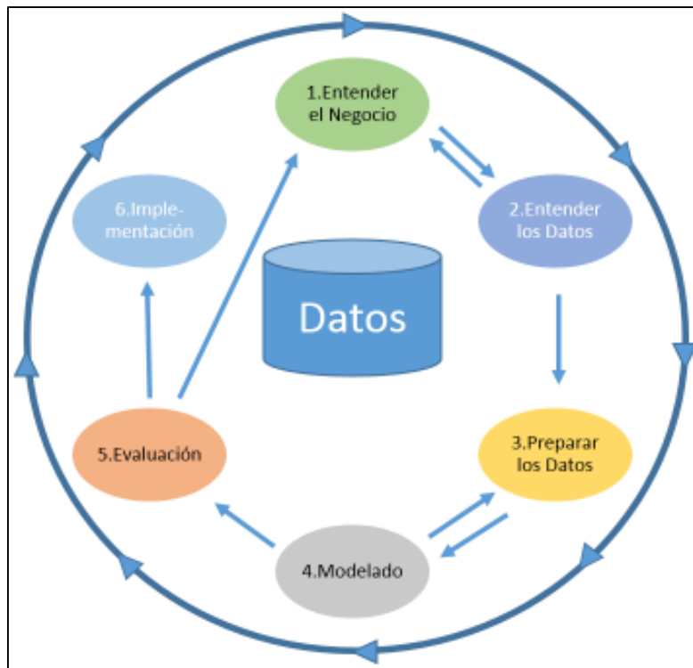
Figura 7: Modelo CRISP-DM
