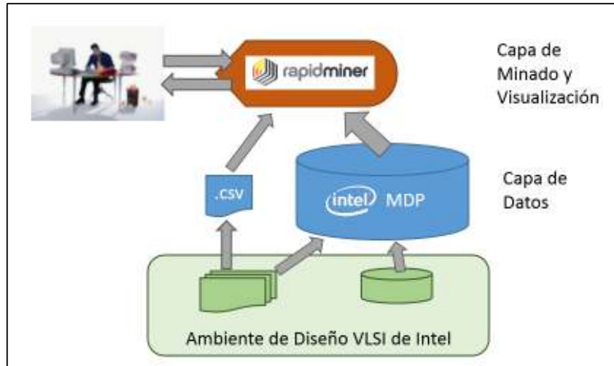
Figura 33: Arquitectura recomendada para el Sistema de Minado de Datos
