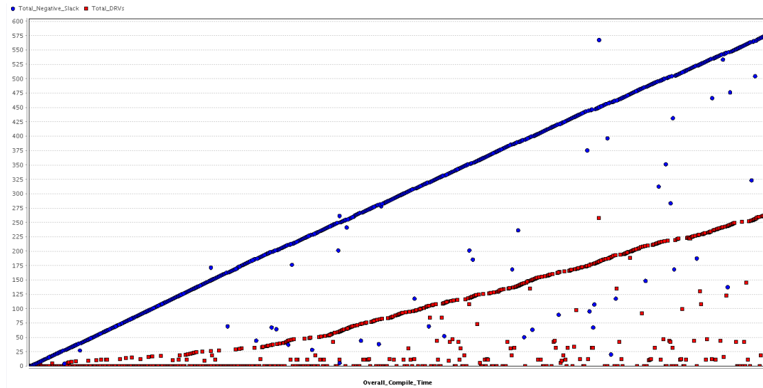
Figura 19: Correlación entre TNS (azul), violaciones a reglas de diseño (rojo) y el tiempo de ejecución
