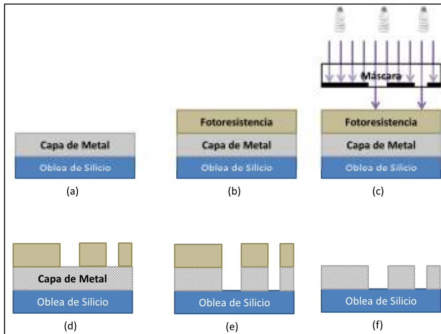
Figura 3: Proceso de fotolitografía
