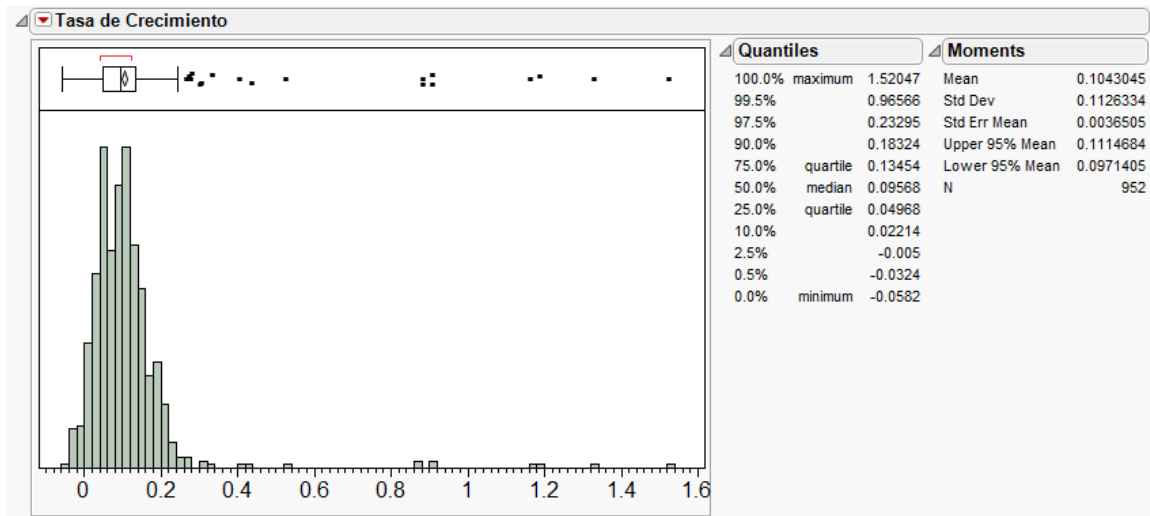
Figura 26: Distribución de tasa de crecimiento de celdas
