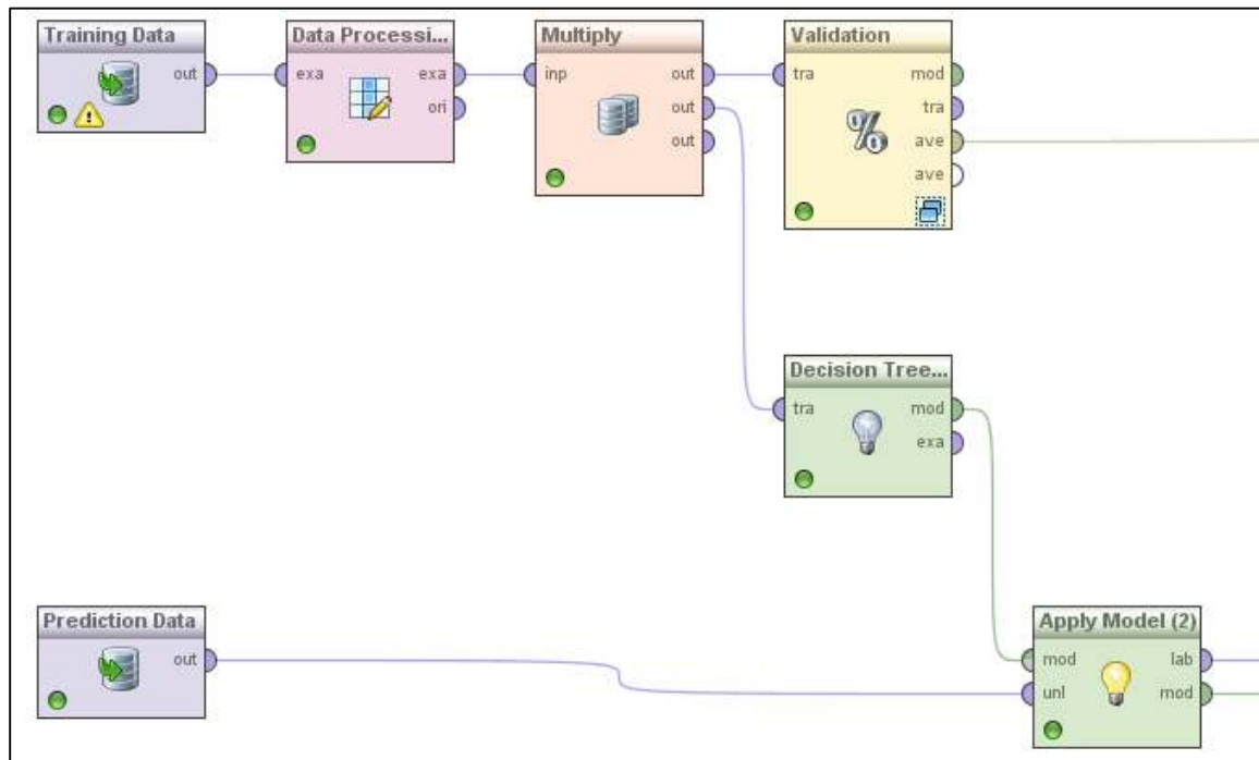
Figura 34: Flujo recomendado de RapidMiner para modelos predictivos
