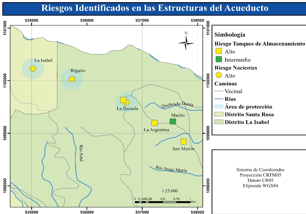
Figura 5.14. Mapa de riesgos SERSA identificados en el acueducto de Alto Varas. Elaborado a partir del Atlas Digital (Tecnológico de Costa Rica, 2014)
