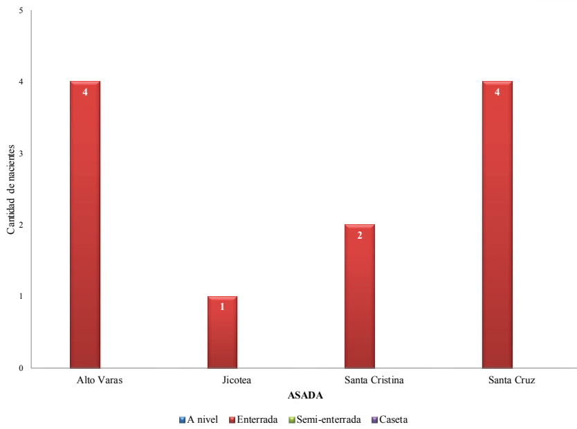
Figura 5.3 Tipo de nacientes en funcionamiento por cada acueducto – Turrialba.
