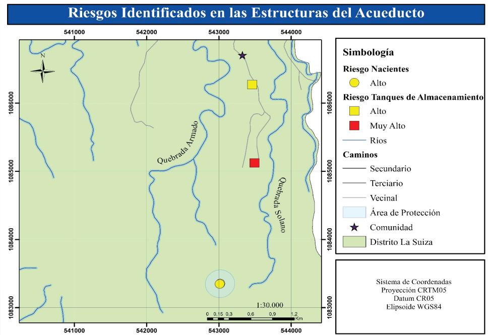
Figura 5.16. Mapa de riesgos SERSA identificados en el acueducto de Santa Cristina. Elaborado a partir del Atlas Digital (Tecnológico de Costa Rica, 2014)
