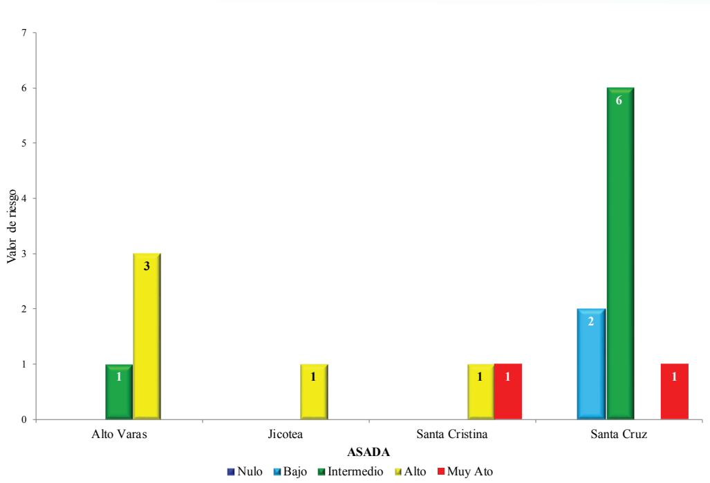
Figura 5.10 Riesgo SERSA para los tanques de almacenamiento de los acueductos – Turrialba.
