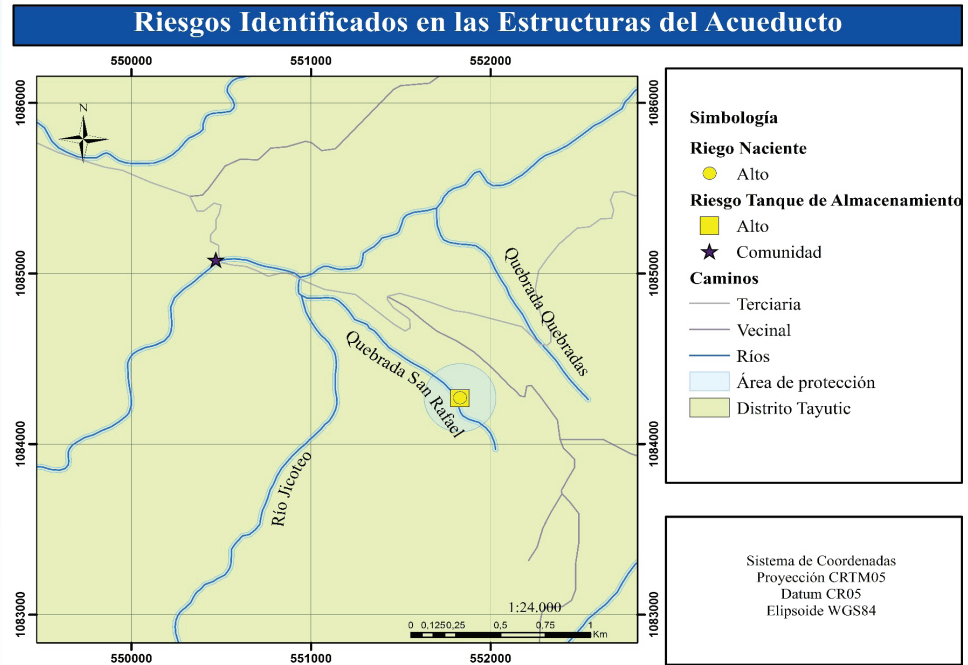
Figura 5.15. Mapa de riesgos SERSA identificados en el acueducto de Jicotea. Elaborado a partir del Atlas Digital (Tecnológico de Costa Rica, 2014)
