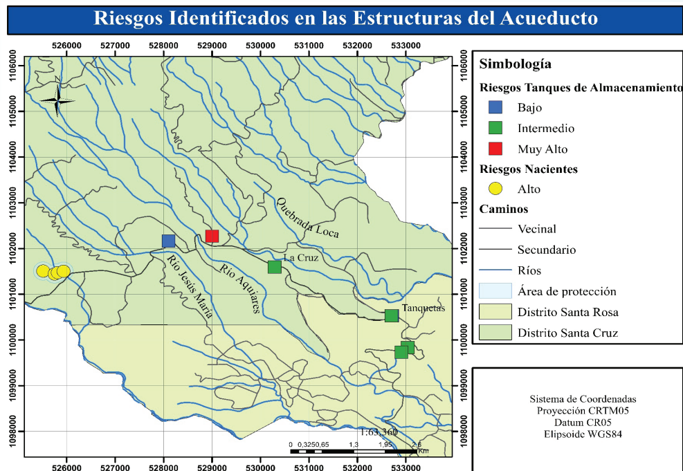
Figura 5.17. Mapa de riesgos SERSA identificados en el acueducto de Santa Cruz. Elaborado a partir del Atlas Digital (Tecnológico de Costa Rica, 2014)
