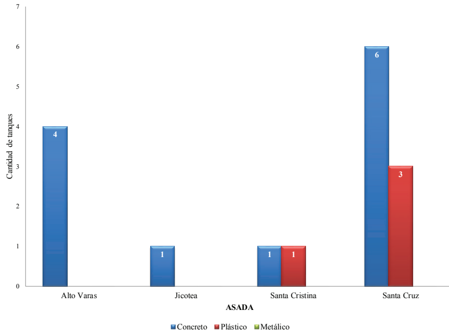
Figura 5.6 Material de los tanques de almacenamiento en funcionamiento por acueducto – Turrialba.
