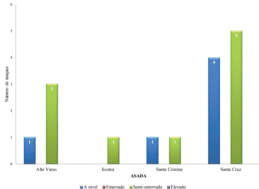
Figura 5.5 Número y tipo de construcción de los tanques de almacenamiento por acueducto – Turrialba.
