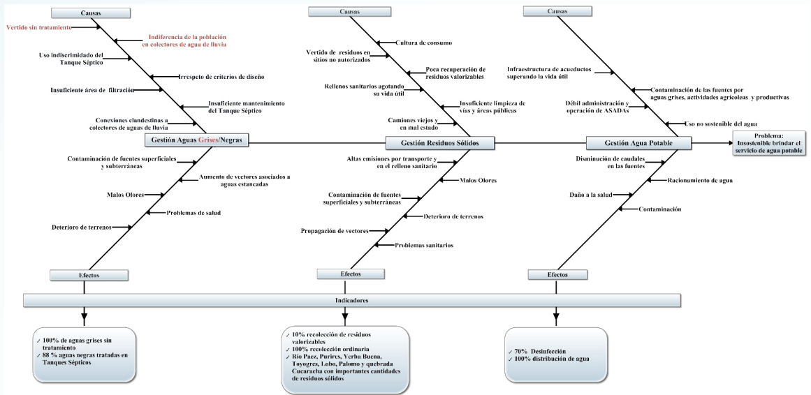
Figura 5.32. Análisis causa - efecto del sistema de agua potable de las ASADAs de la Provincia de Cartago.
