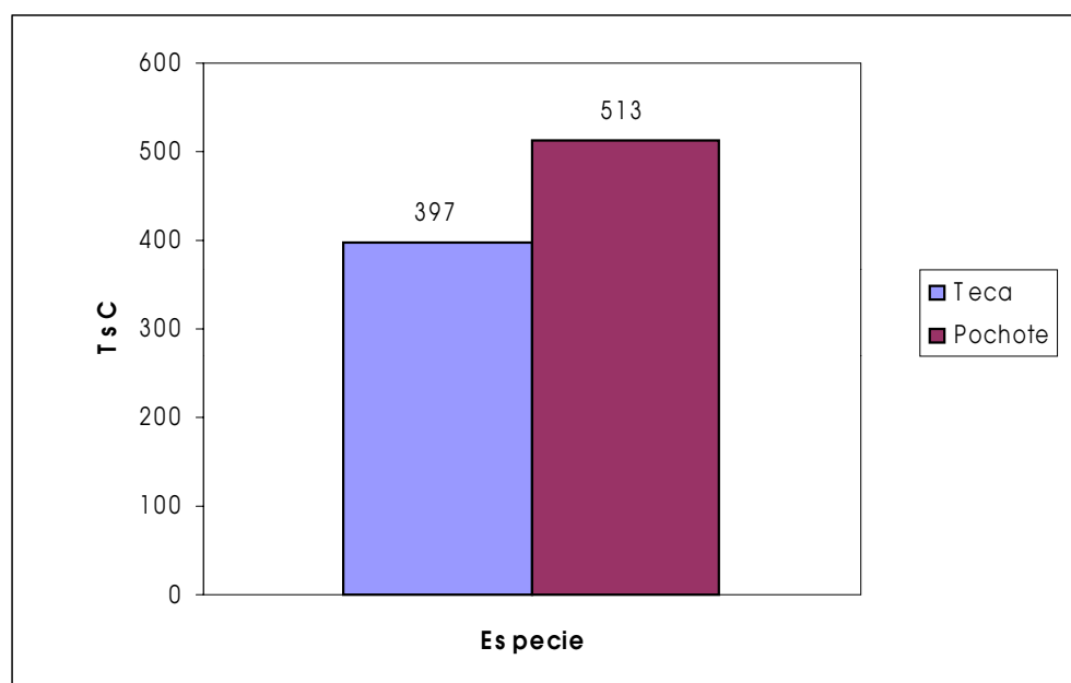
Figura 17. Promedio general de las TsC para Teca ( Tectona grandis ) y Pochote ( Bombacopsis quinatum ). Guanacaste, 2001.
