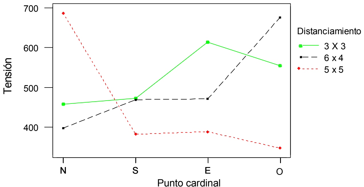
Figura 15. Interacción de los Puntos Cardinales con los tres distanciamientos de siembra (3 x 3 m, 5 x 5 m y 6 x 4 m) para Pochote ( Bombacopsis quinatum ) en los Proyectos Forestales Garza y Río Tabaco. Guanacaste, 2001.
