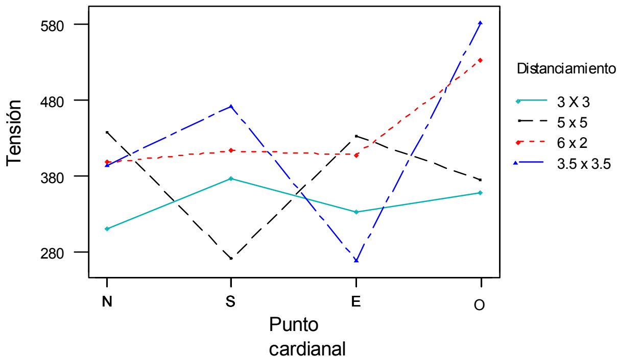
Figura 11. Interacción de los puntos cardinales en los cuatro distanciamientos de siembra evaluados ( 3 x 3 m, 6 x 2 m, 3,5 x 3,5 m y 5 x 5 m) para Teca ( Tectona grandis ), en los Proyectos Forestales Río Tabaco y Garza. Guanacaste, 2001.
