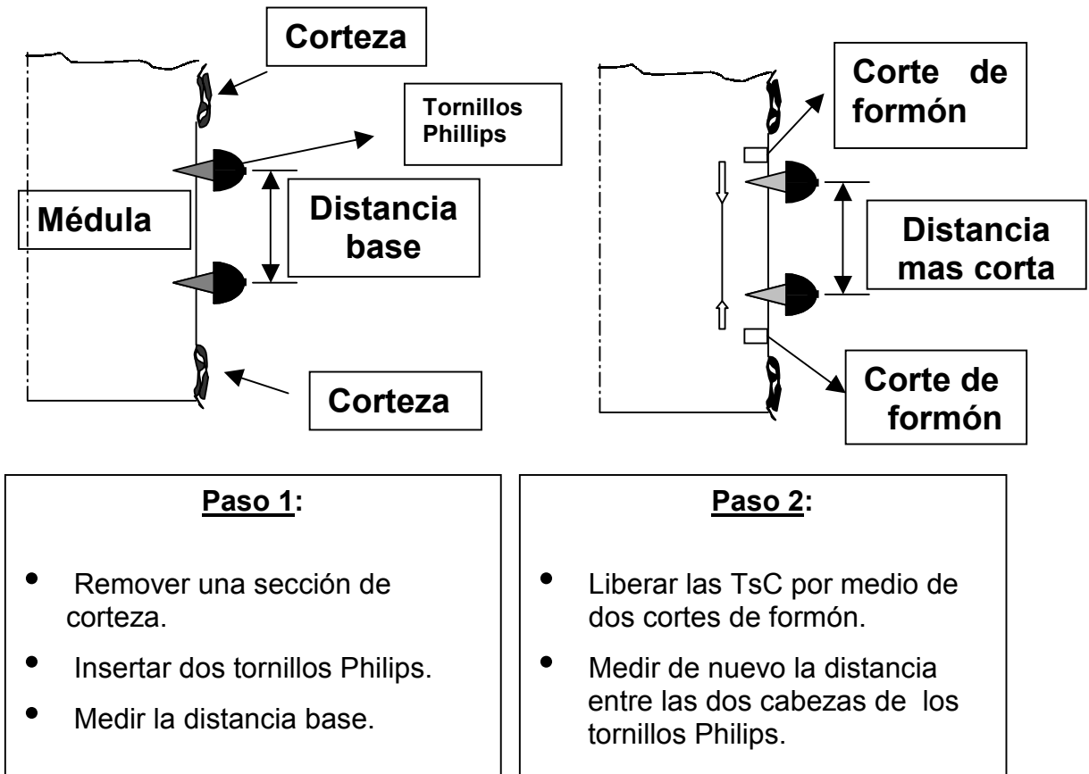
Figura 2. Representación esquemática para medir las deformaciones unitarias a causa de la liberación de las tensiones de crecimiento (TsC).
