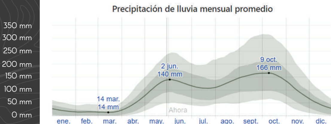
Gráfico 8: Precipitación Fuente: Elaboración Propia, en base a Climate Consultant
