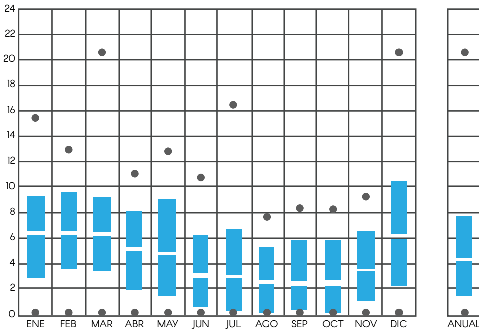
Gráfico 10: Velocidad de los vientos Fuente: Elaboración Propia, en base a Climate Consultant
