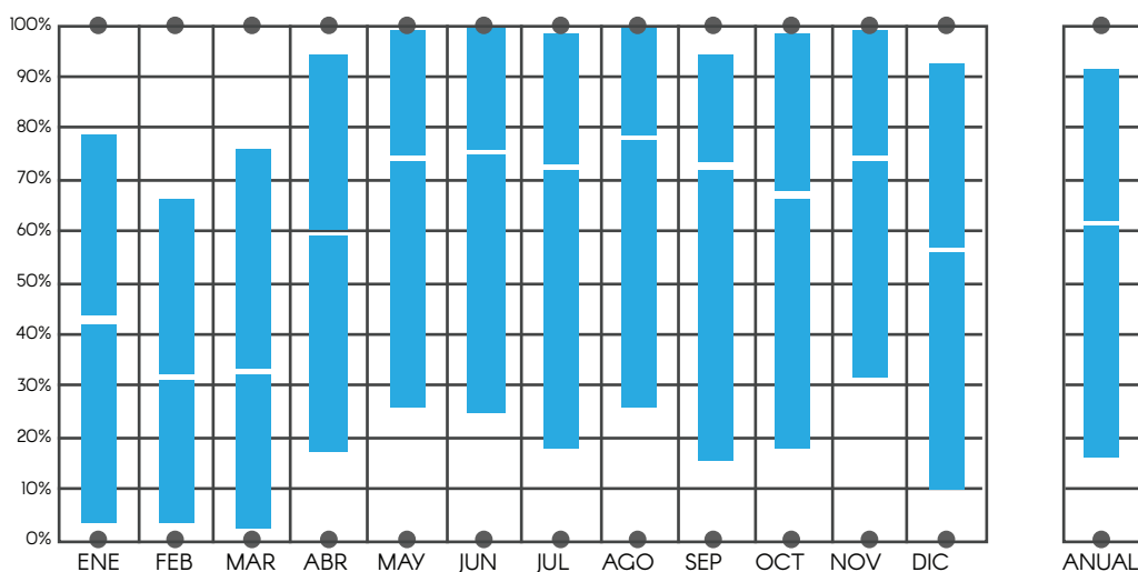
Gráfico 13: Cobertura de nubes Fuente: Elaboración Propia, en base a Climate Consultant
