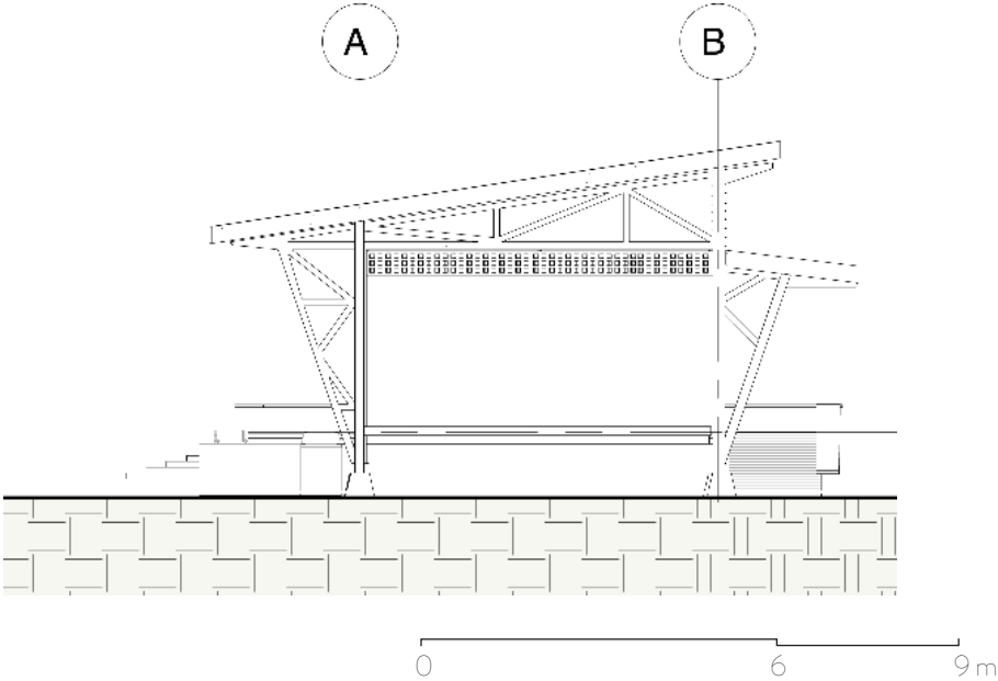
Figura 4.53: Elevaciones Bloque D Fuente:Elaboración propia
