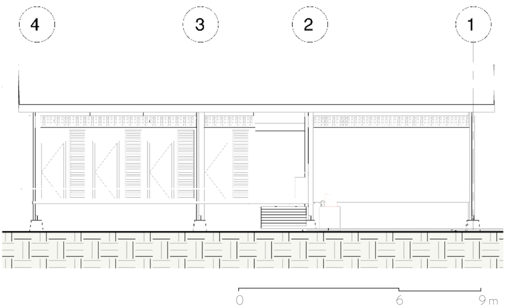
ELEVACIÓN POSTERIOR
