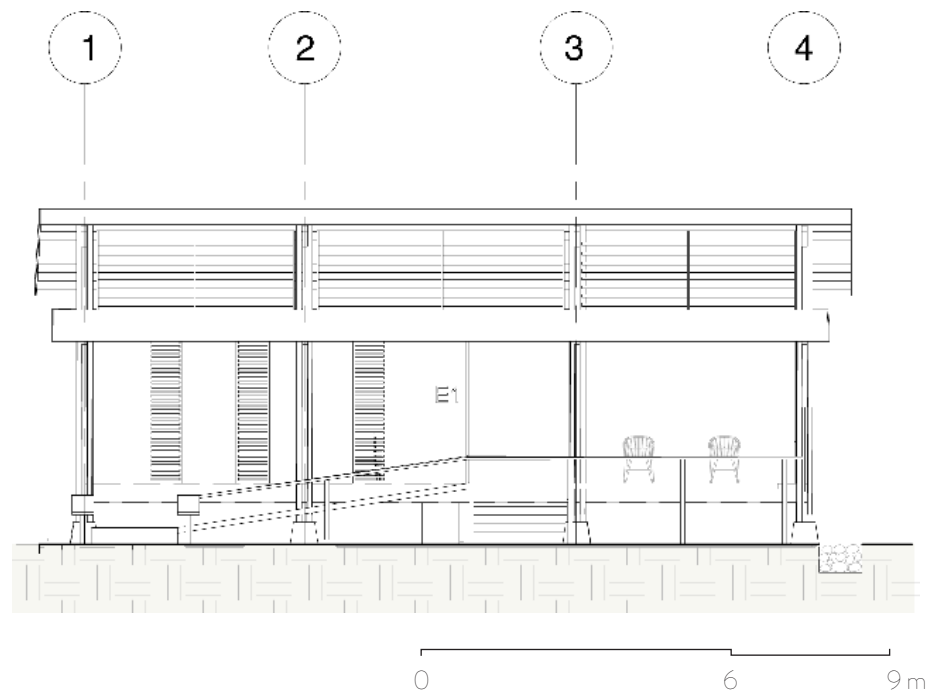
ELEVACIÓN FRONTAL
