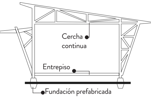
Figura 4.21: Módulo de Sección típica Fuente:Elaboración propia
