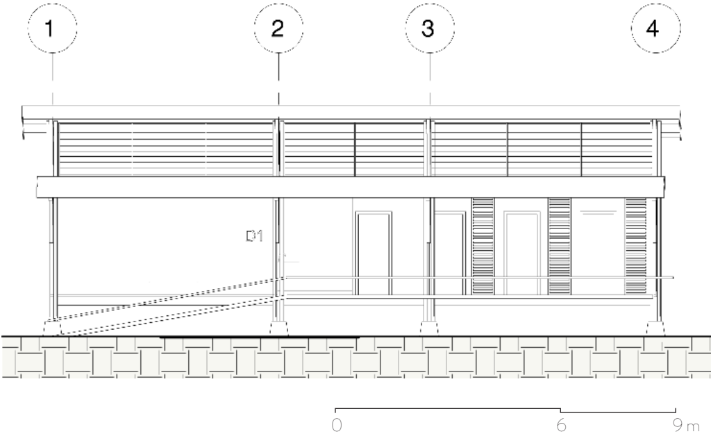
ELEVACIÓN FRONTAL
