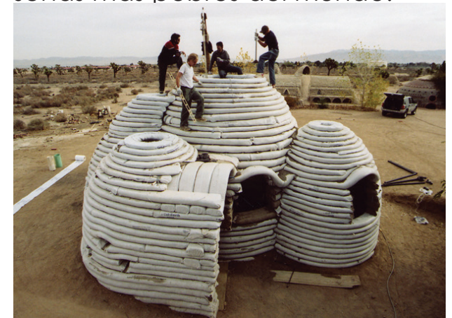
imagen # 47 construccion en superadobe
