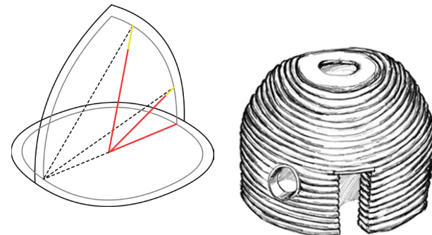
imagen # 48 esquema básico superadobe y su uso en la exploración espacial
