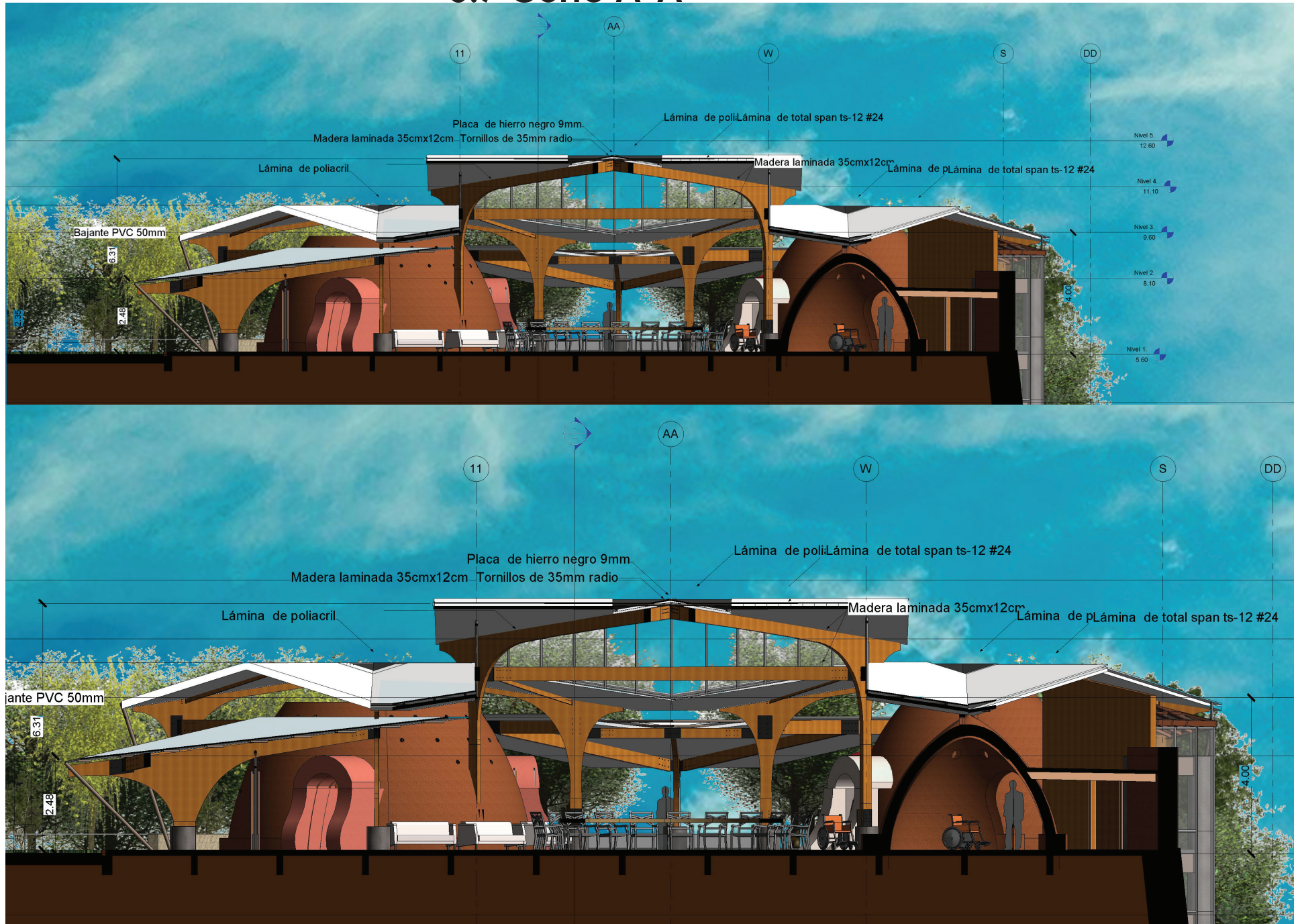
imagen #79 Corte A-A'
