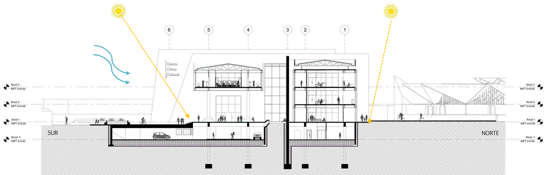
CORTE B-B
