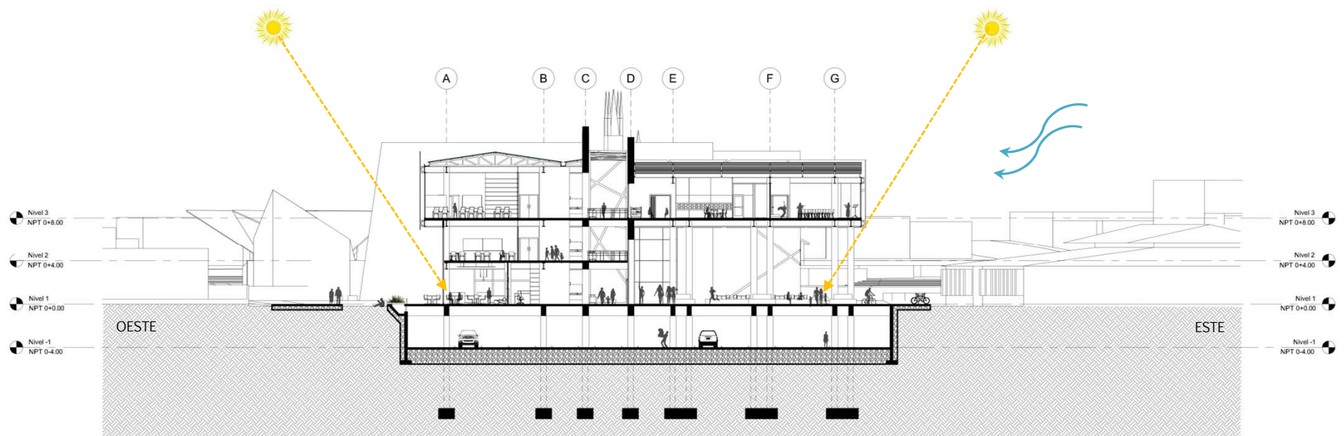
CORTE A-A
