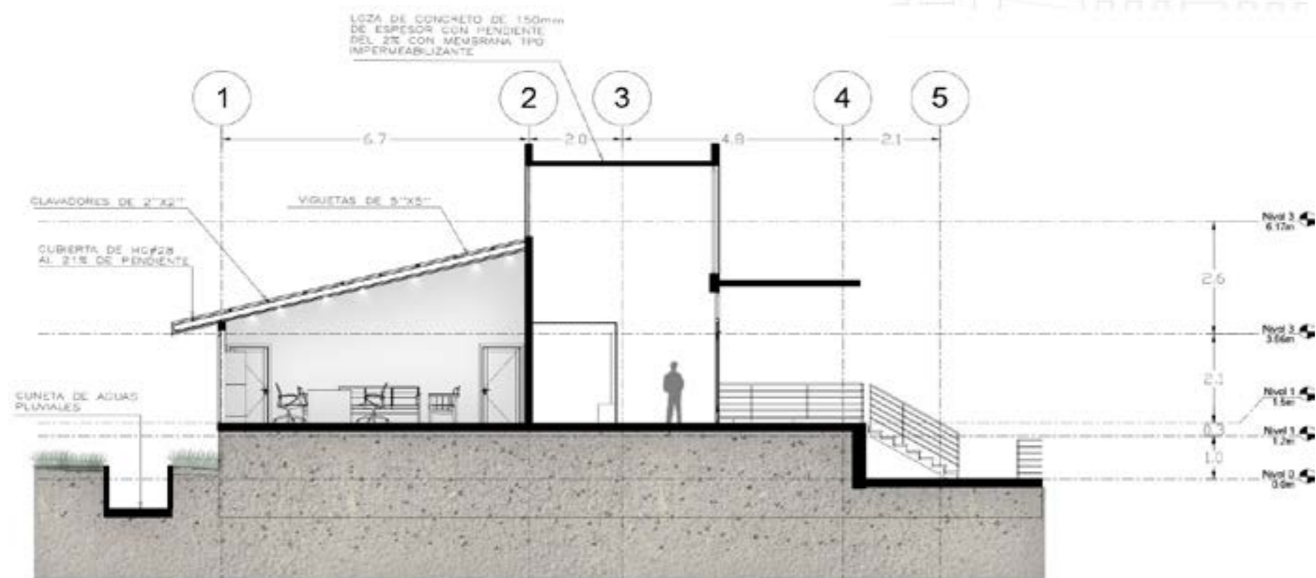
Imagen 272 - Sección A-A
