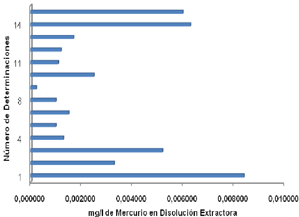
Figura 8. Determinación del Mercurio en la Disolución Extractora por Espectroscopia de Absorción Atómica.
