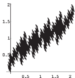
Figura 2.2 Fracciones con b = 2 - i
