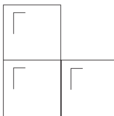
Figura 4.7 MCRM cuyo atractor es el Triángulo de Sierpiński.
