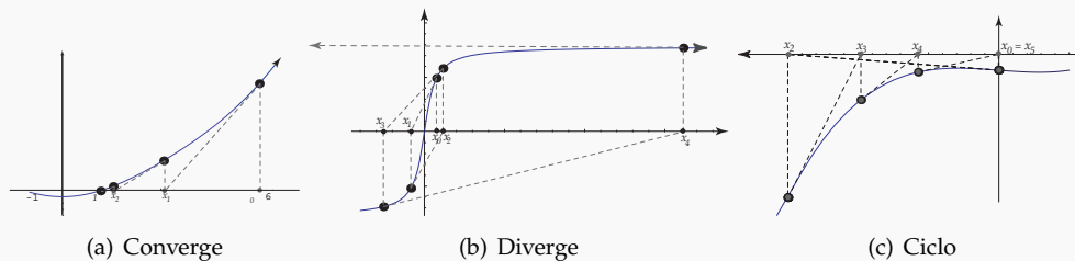
Figura 6.3 Iteración de Newton
