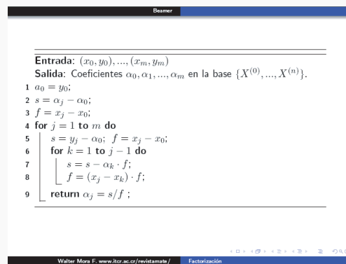
Figura 10.12 Beamer con algorithm2e
