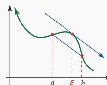
Figura 6.2 Teorema del valor medio
