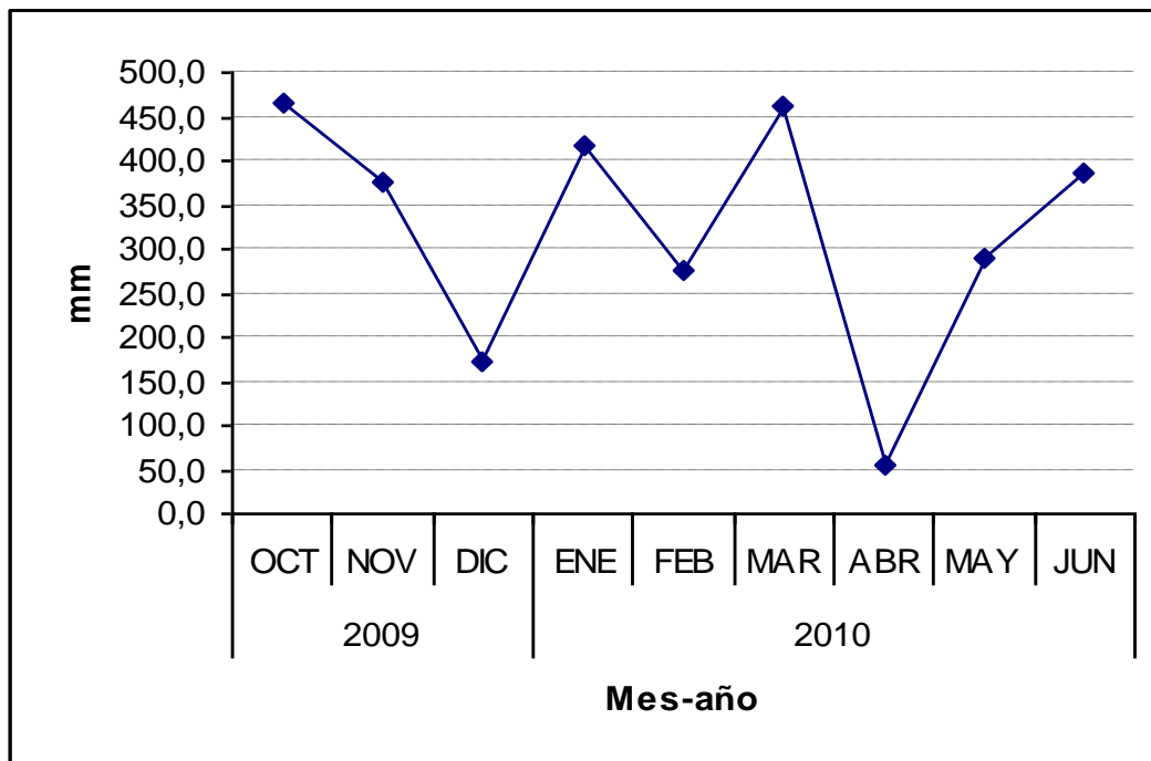
Figura 5. Comportamiento de la precipitación (mm), durante el periodo del experimento, Finca El Tremedal S.A. Venecia, San Carlos, Costa Rica. 2009-2010.
