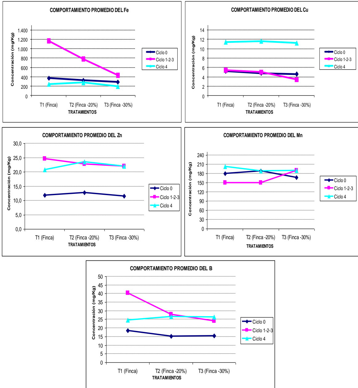
Figura 11. Concentración de microelementos en los análisis foliares en plantas de piña ( Ananas comosus ) (L.) Merr híbrido MD-2, fertilizados mediante el Método Stroller. Finca El Tremedal S.A. Venecia, San Carlos, Costa Rica. 2010.
