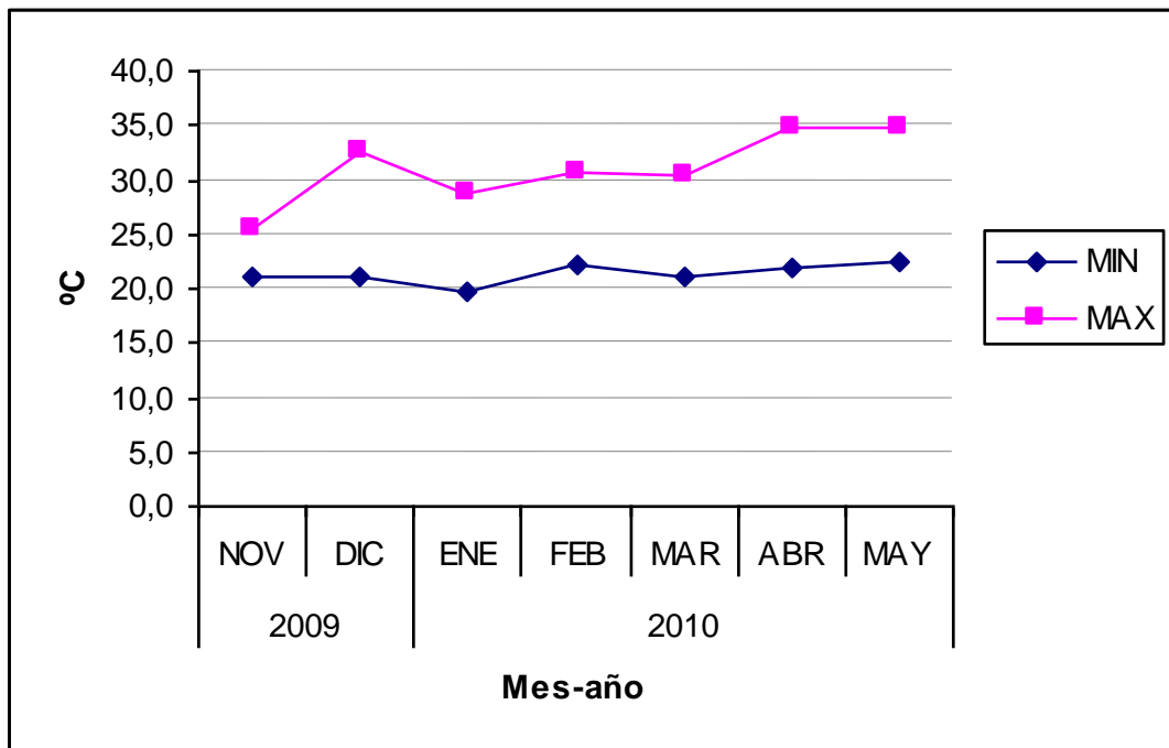
Figura 6. Comportamiento de la temperatura, durante el periodo del experimento, Finca El Tremedal S.A. Venecia, San Carlos, Costa Rica. 2009-2010.
