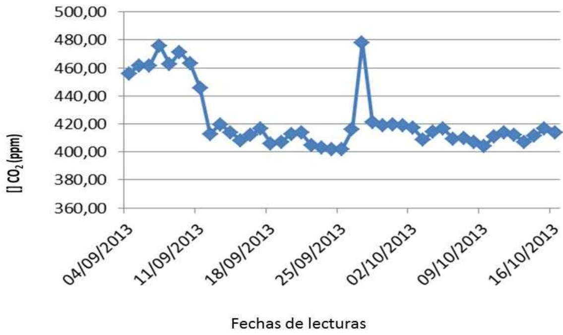
Concentración de dióxido de carbono en el ambiente protegido donde se desarrolló ensayo, datos para siembra 4
