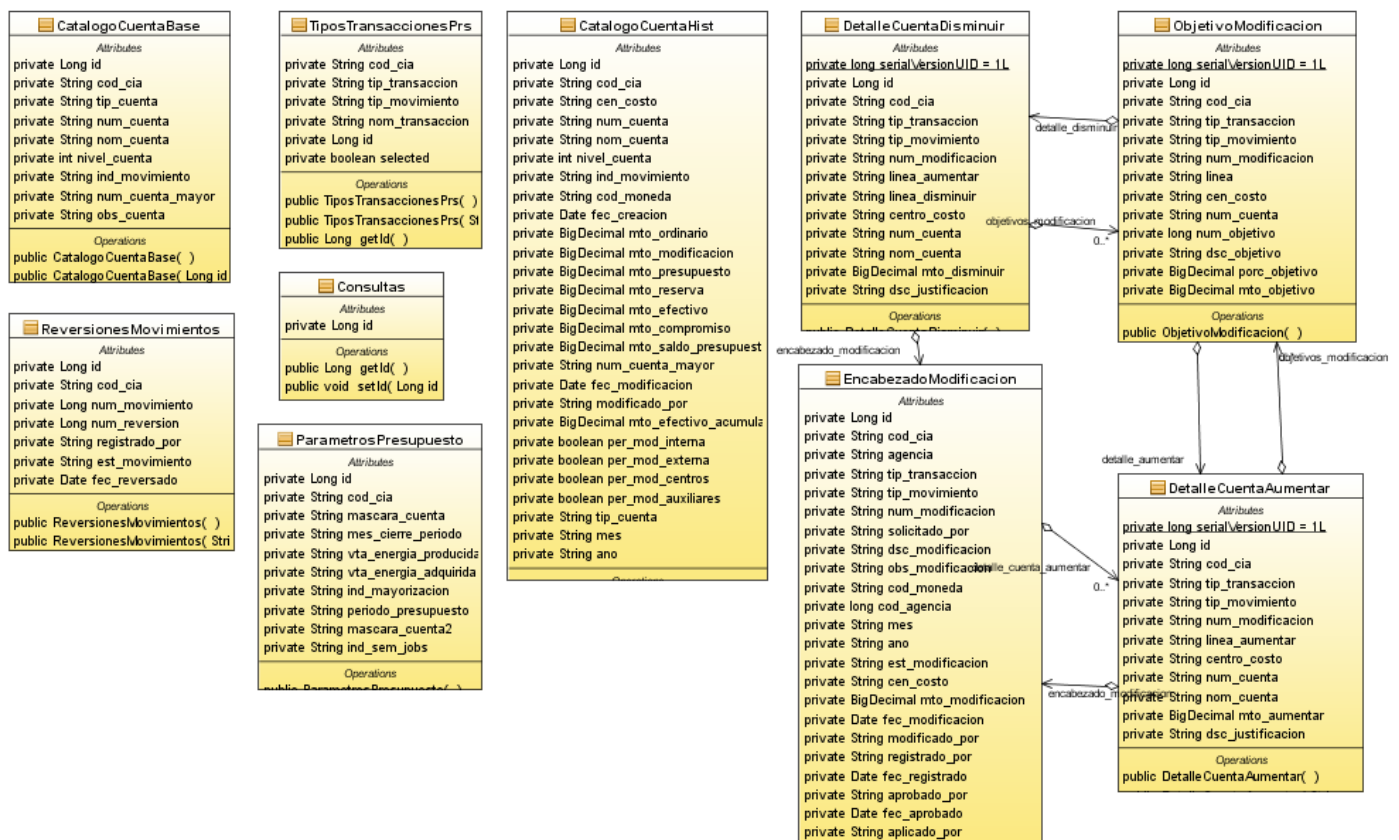
Ilustración 3 - Muestra el diagrama de clases del módulo de presupuesto 1.
