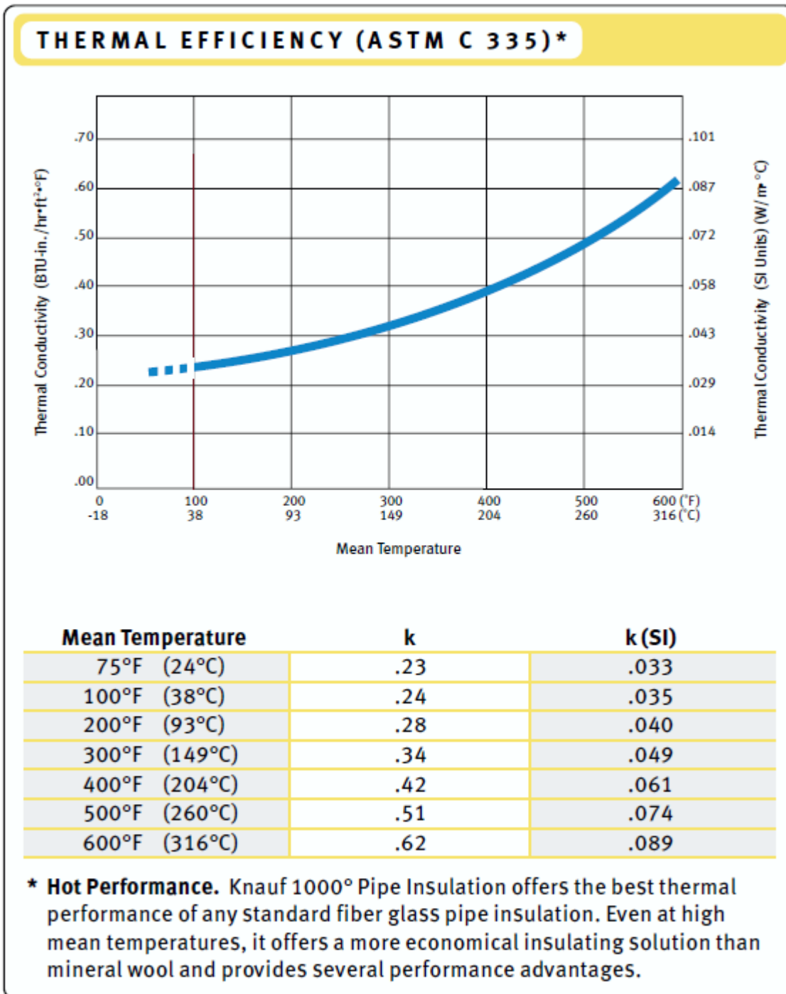
Figura 10.11. Conductividad del aislamiento según temperatura media.
