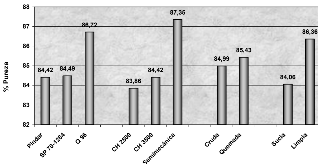
Figura 16. Porcentaje de Pureza del jugo para los diferentes factores evaluados en el estudio de Materia Extraña. Ingenio Quebrada Azul, San Carlos, 2005.
