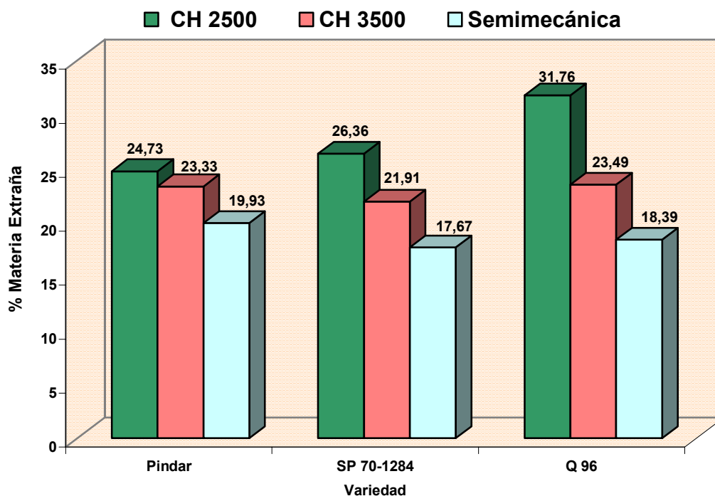
Figura 6. Contenidos (%) de Materia Extraña presentes según Variedad Cultivada vs Tipo de Cosecha evaluada, Ingenio Quebrada Azul, San Carlos, 2005.
