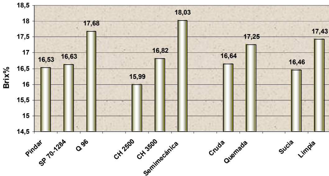
Figura 10. Porcentaje de Brix para los diferentes factores evaluados en el Estudio de Materia Extraña, Ingenio Quebrada Azul, San Carlos, 2005.
