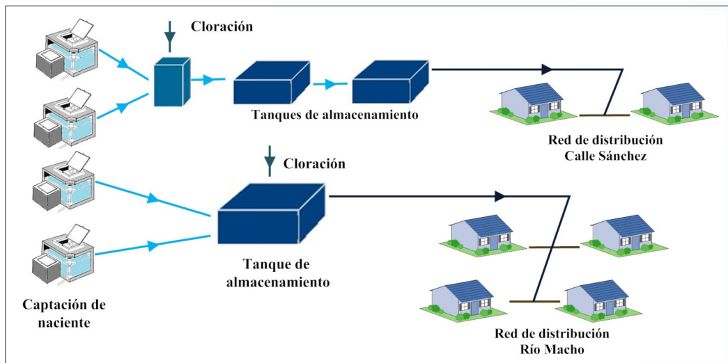
Figura 3.1. Esquema del sistema del acueducto de Río Macho
