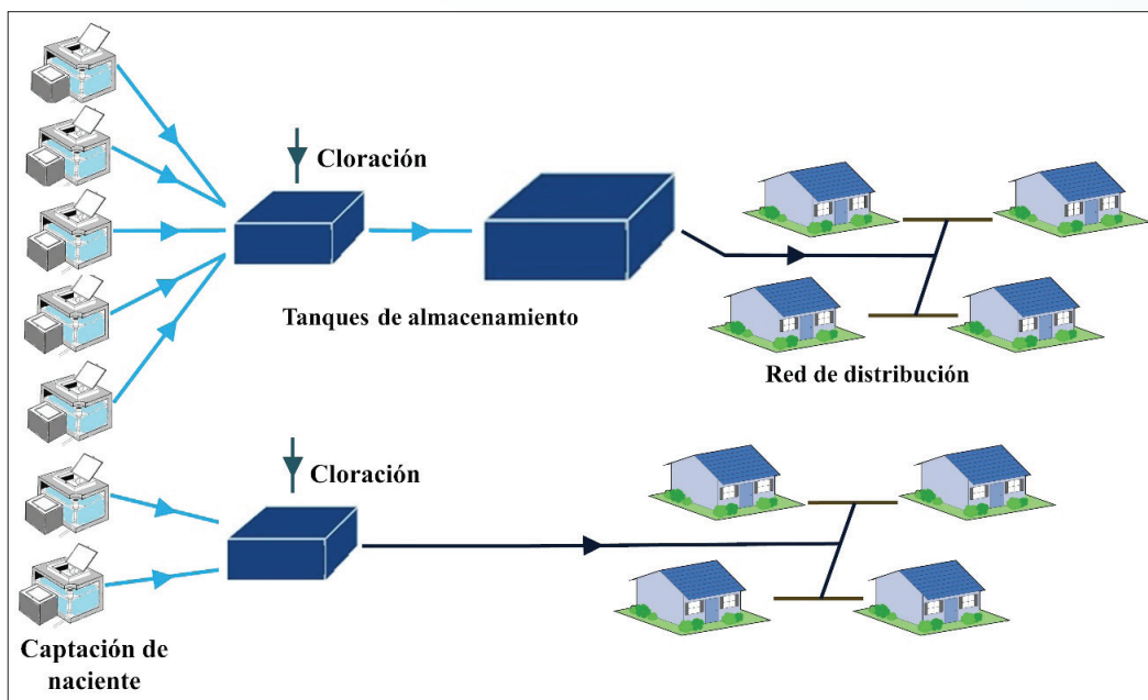
Figura 3.1. Esquema del sistema del acueducto de Cot.
