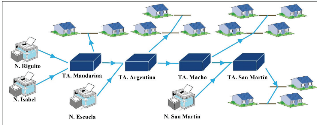
Figura 3.1. Esquema del sistema del acueducto de Alto Varas.
