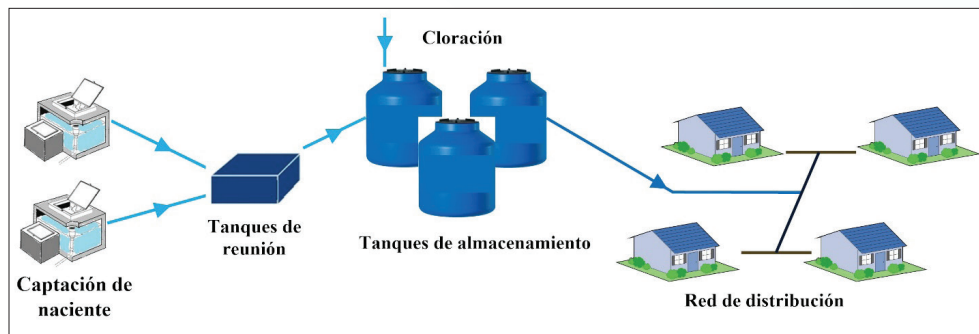
Figura 3.1. Esquema del sistema del acueducto de Cooperosales.
