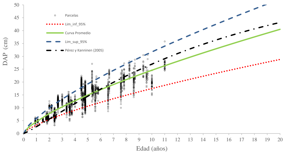
Figura 7. Índice de sitio superior del modelo de crecimiento de teca a partir de semilla (Pérez y Kanninen 2005) vs el modelo clonal ajustado para teca en esta investigación en Costa Rica.
